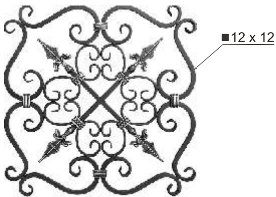
40115 470 x 470 mm 6,1 kg
