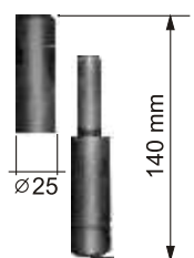
30051 \varnothing 25 x 140 mm 0,52 kg
