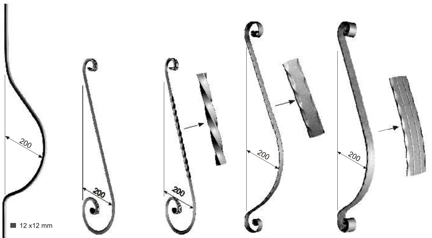
h = 750 mm ■ 12 75030 1,45 kg ■ 14 75230 2,26 kg
