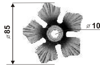
64022 85 x 85 x 1,5 mm 0,05 kg
