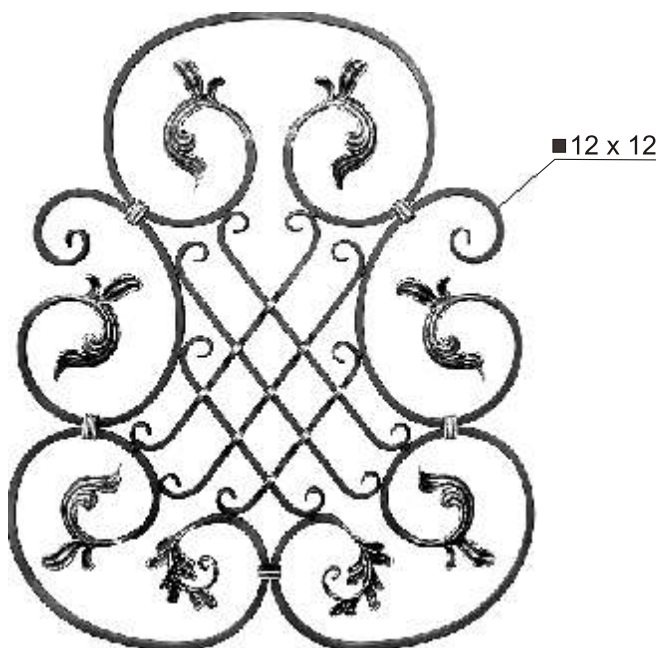
40117 700 x 850 mm 9,5 kg
