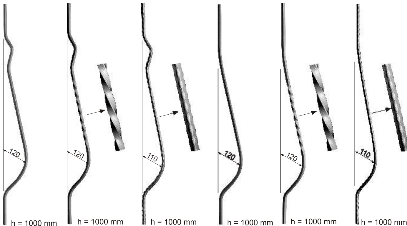
h = 1000 mm ■ 12 75010 1,22 kg ■ 14 75210 1,79 kg
