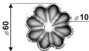
64005.06 60 x 60 x 2 mm 0,05 kg
